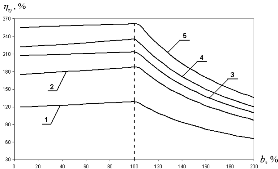
Рис. 4. Графік залежності КВЕ ТНСУ з байпасуванням від коефіцієнта теплових втрат: 1 – при \varphi_{cm} = 50 \% ; 2 – \varphi_{cm} = 60 \% ; 3 – \varphi_{cm} = 70 \% ; 4 – \varphi_{cm} = 80 \% ; 5 – \varphi_{cm} = 90 \%
