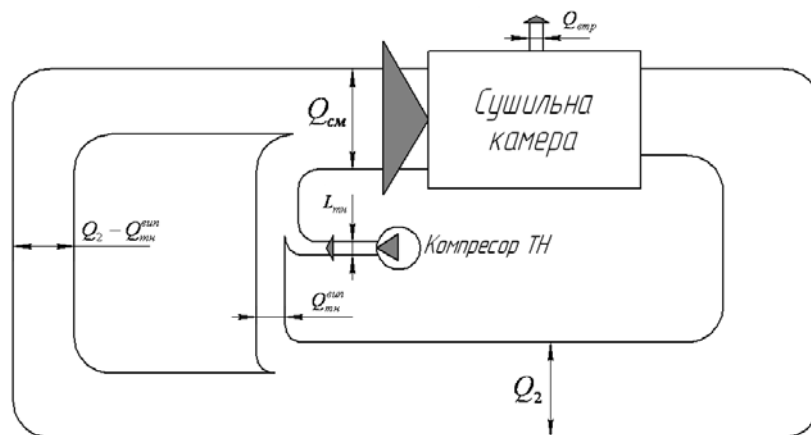
Рис. 2. Діаграма потоків енергії ТНСУ при K=1
